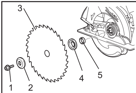
► 1. Tornillo hexagonal 2. Brida exterior 3. Disco de sierra 4. Brida interior 5. Anillo de ajuste
