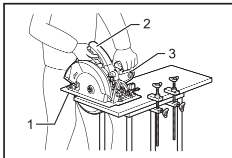
► 1. Base 2. Poignée arrière 3. Poignée avant
