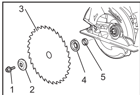
► 1. Boulon hexagonal 2. Bague externe 3. Lame 4. Bague interne 5. Bague
