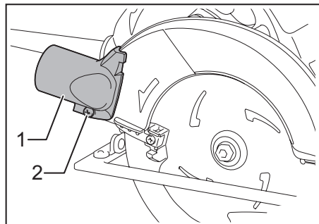
► 1. Raccord à poussières 2. Vis
