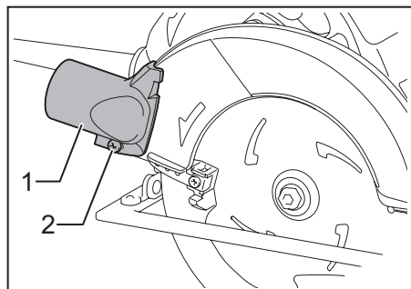
► 1. Boquilla para polvo 2. Tornillo
